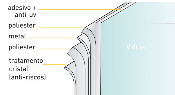
COMPOSIÇÃO DA PELÍCULA (ARGENT 80C)
