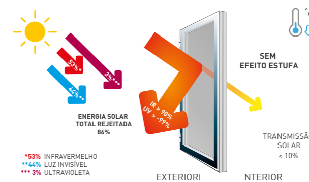
VIDRO SIMPLES COM O SILVER 285XC
