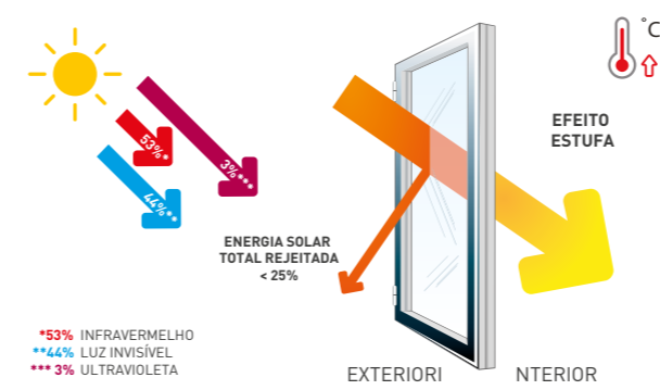
VIDRO SIMPLES SEM PELÍCULA
